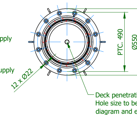
A-A (1:20)
